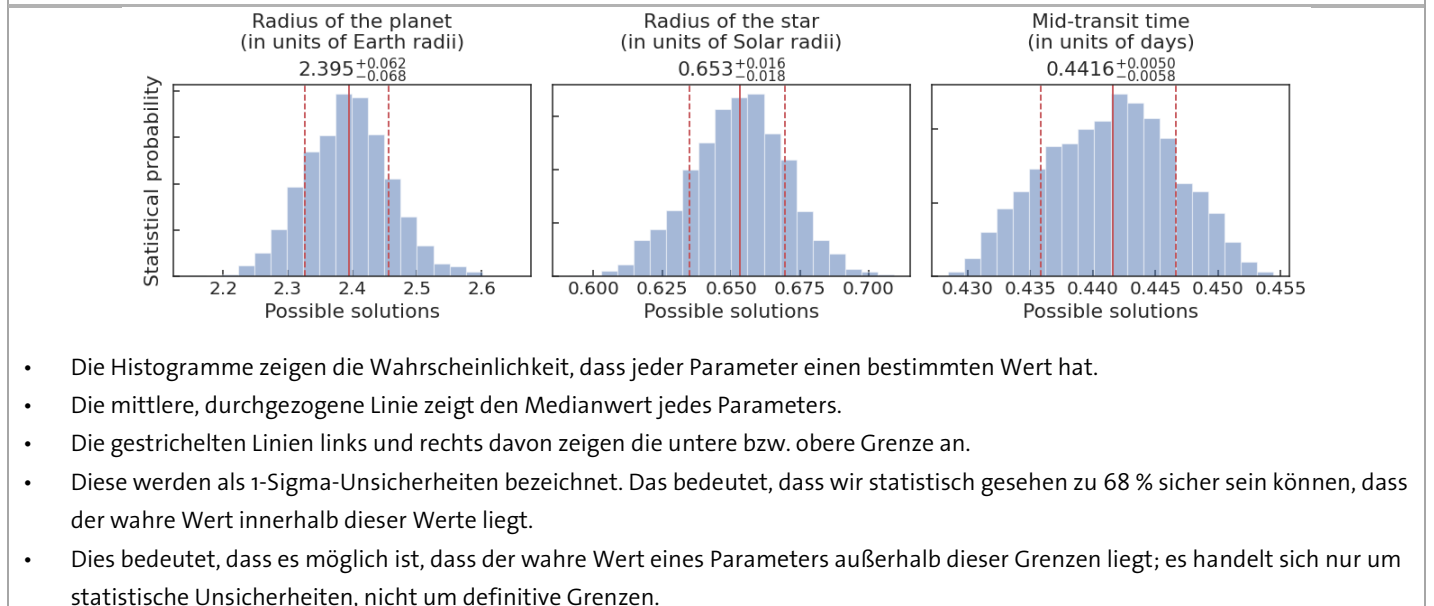
↑ Histogramm der statistischen Wahrscheinlichkeit für alle Parameterwerte des TOI-560c
